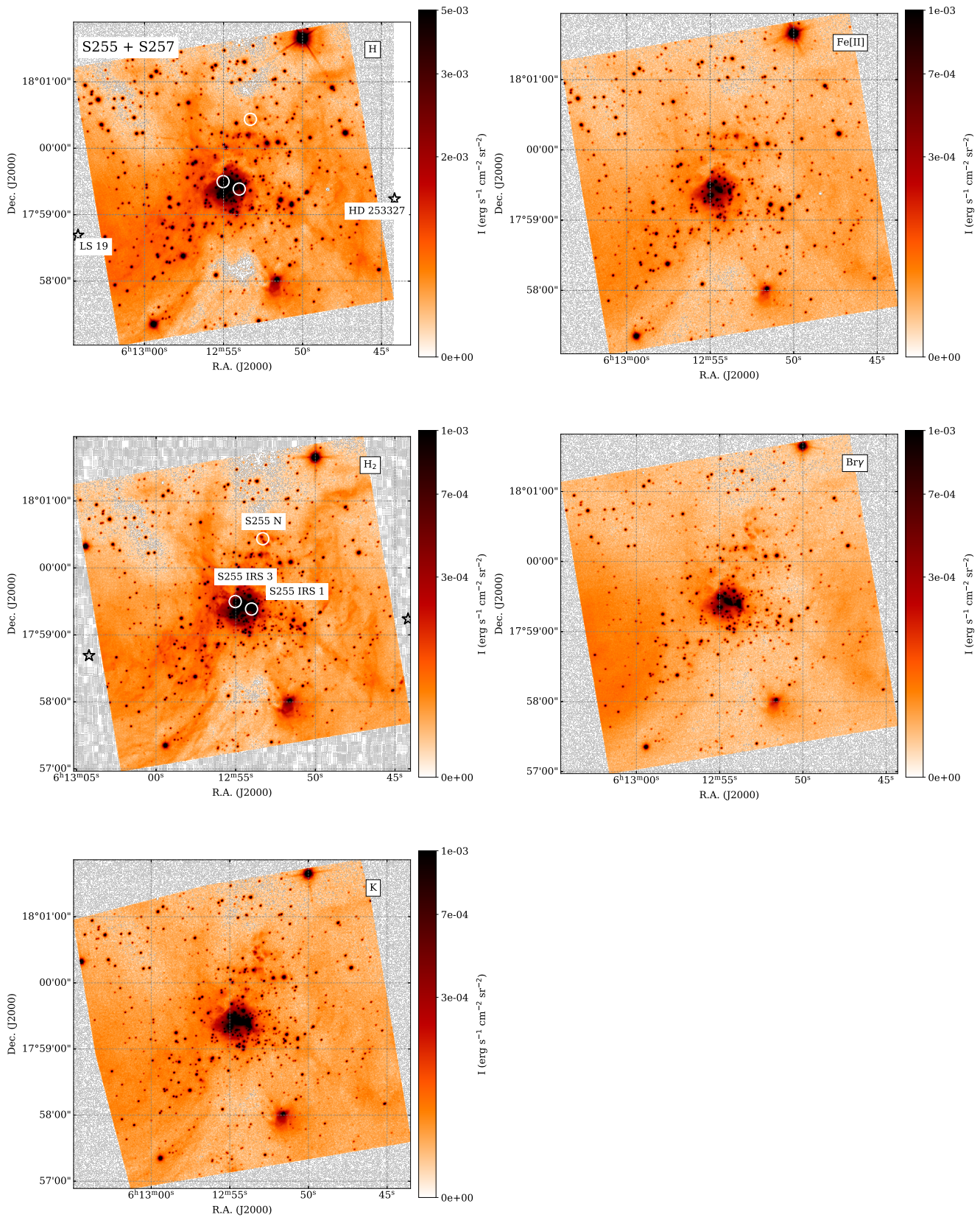
Рис. 3. То же, что на рис. 1, для ФДО S255-S257.
