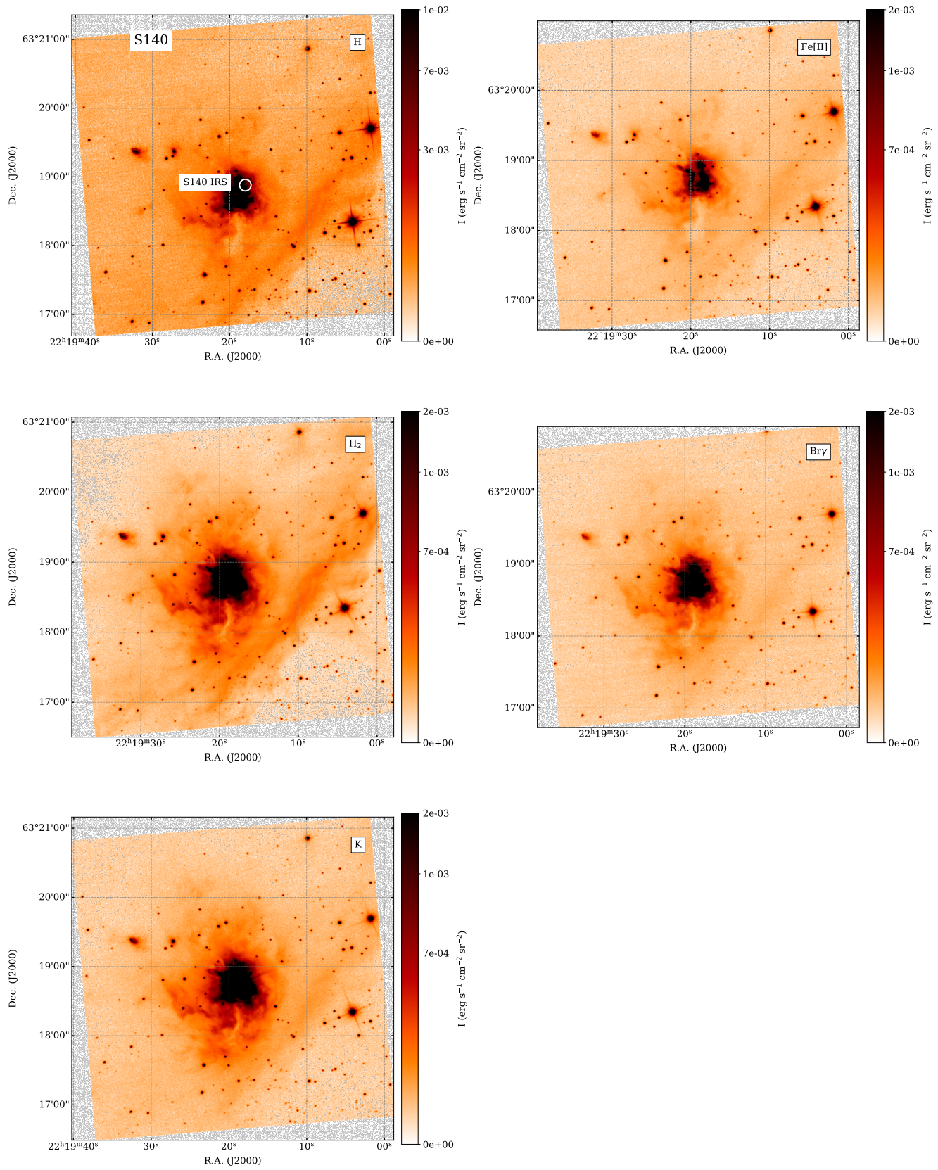
Рис. 4. То же, что на рис. 1, для ФДО S140.
