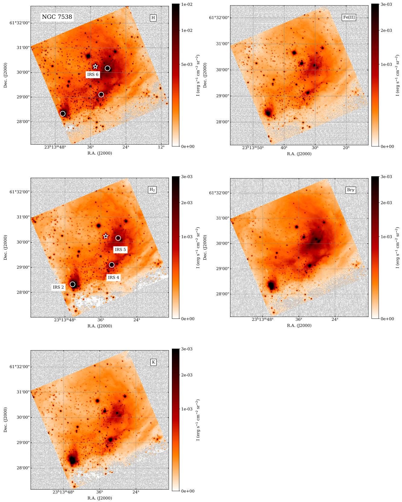
Рис. 2. То же, что на рис. 1, для ФДО NGC 7538.
