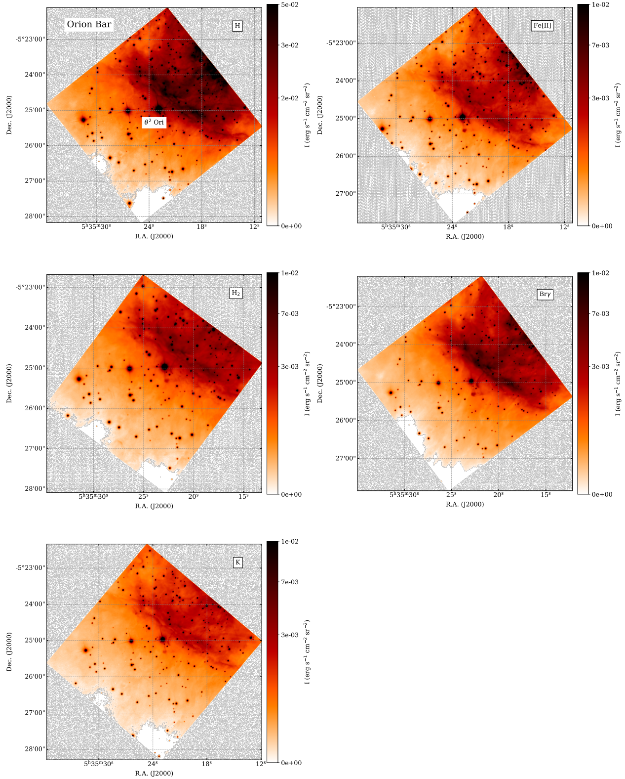
Рис. 1. Откалиброванные по потоку изображения ФДО Перемычка Ориона в использованных в работе фильтрах до вычитания континуума из изображений в фильтрах Br \gamma , [Fe II] и H 2 .
